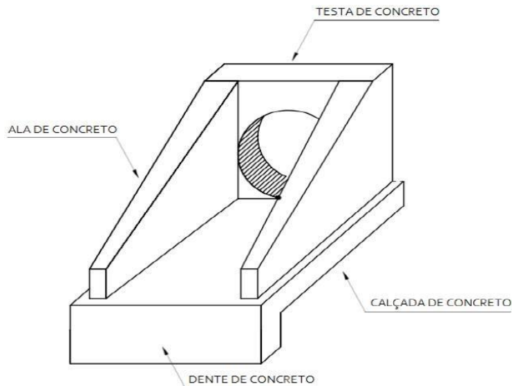
Figura 6 - Boca de bueiro tubular de concreto
