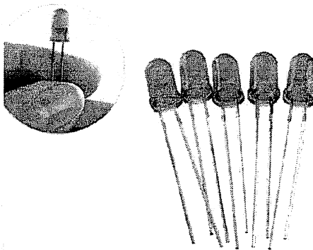
LED Difuso Verde, diâmetro 5mm, tensão de 2V e corrente elétrica de 20 mA.
