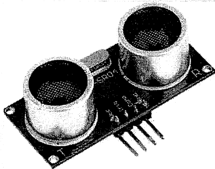
SENSOR ULTRASSÔNICO HC-SR04
