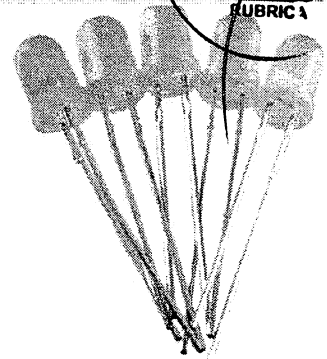
LED Difuso Amarelo, diâmetro 5 mm, tensão de 2 V e corrente elétrica de 20 mA.
