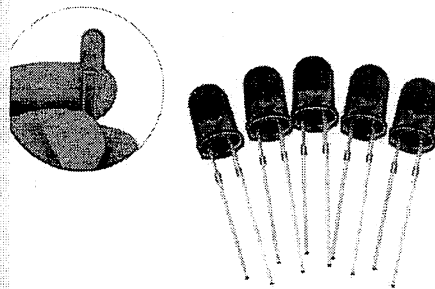
LED Difuso Azul, diâmetro 5 mm, tensão de 2 V e corrente elétrica de 20 mA.
